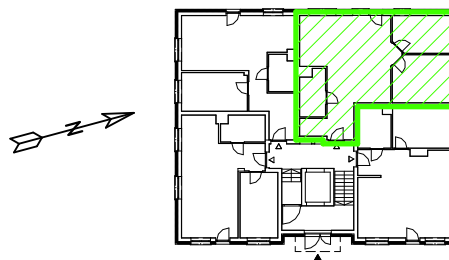
RZUT MIESZKANIA skala 1:100
